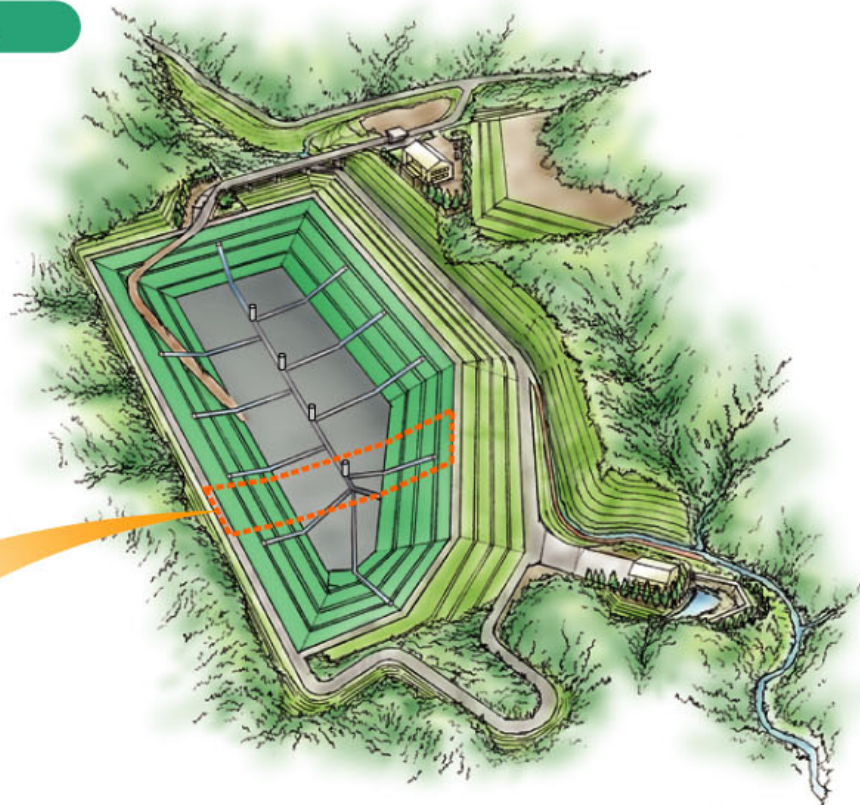
遮水構造イメージ図
