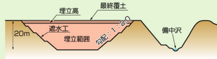
埋立地の基本形状図
