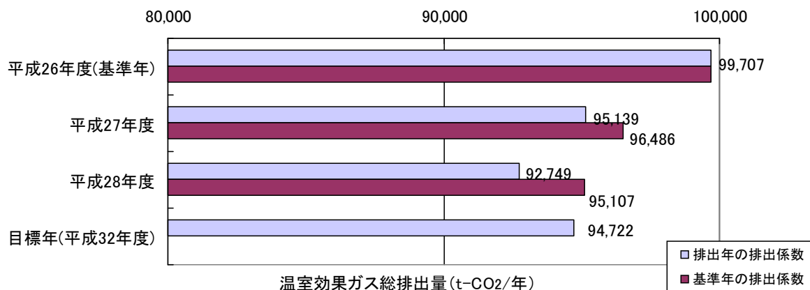
図3-3-1 温室効果ガス総排出量
