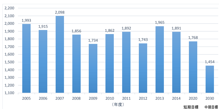
図 3-2-1 温室効果ガス総排出量の推移
