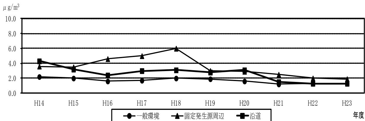
ジクロロメタン濃度の推移〔年平均値〕
