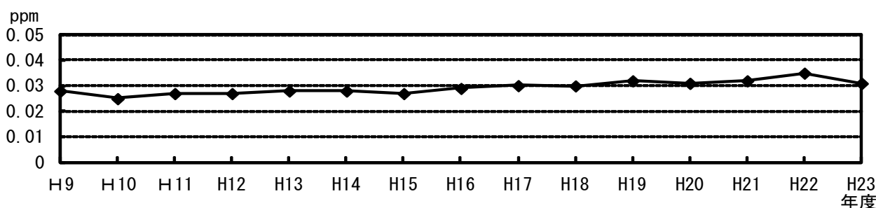
光化学オキシダント濃度の推移〔昼間の1時間値の年平均値〕
