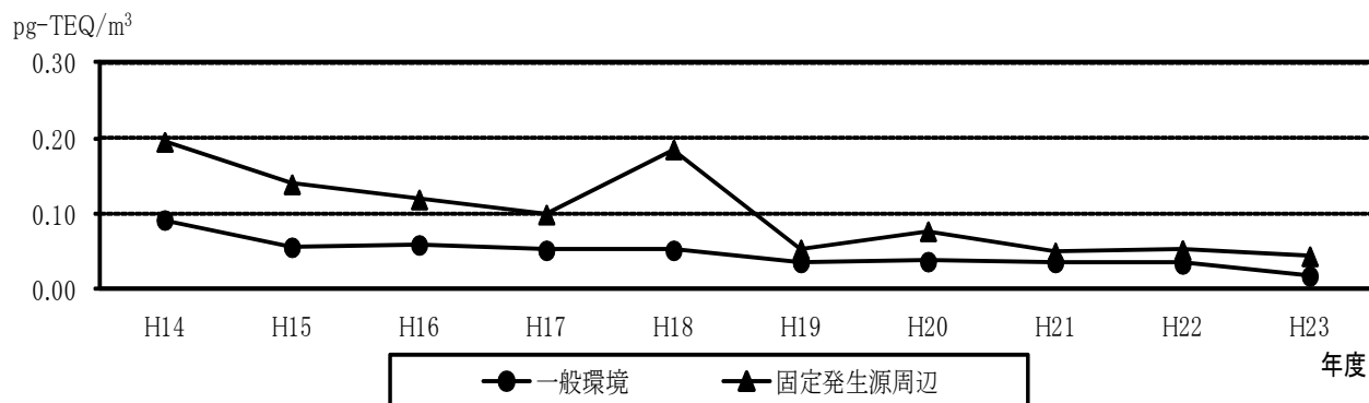
ダイオキシン類濃度の推移〔年平均値〕
