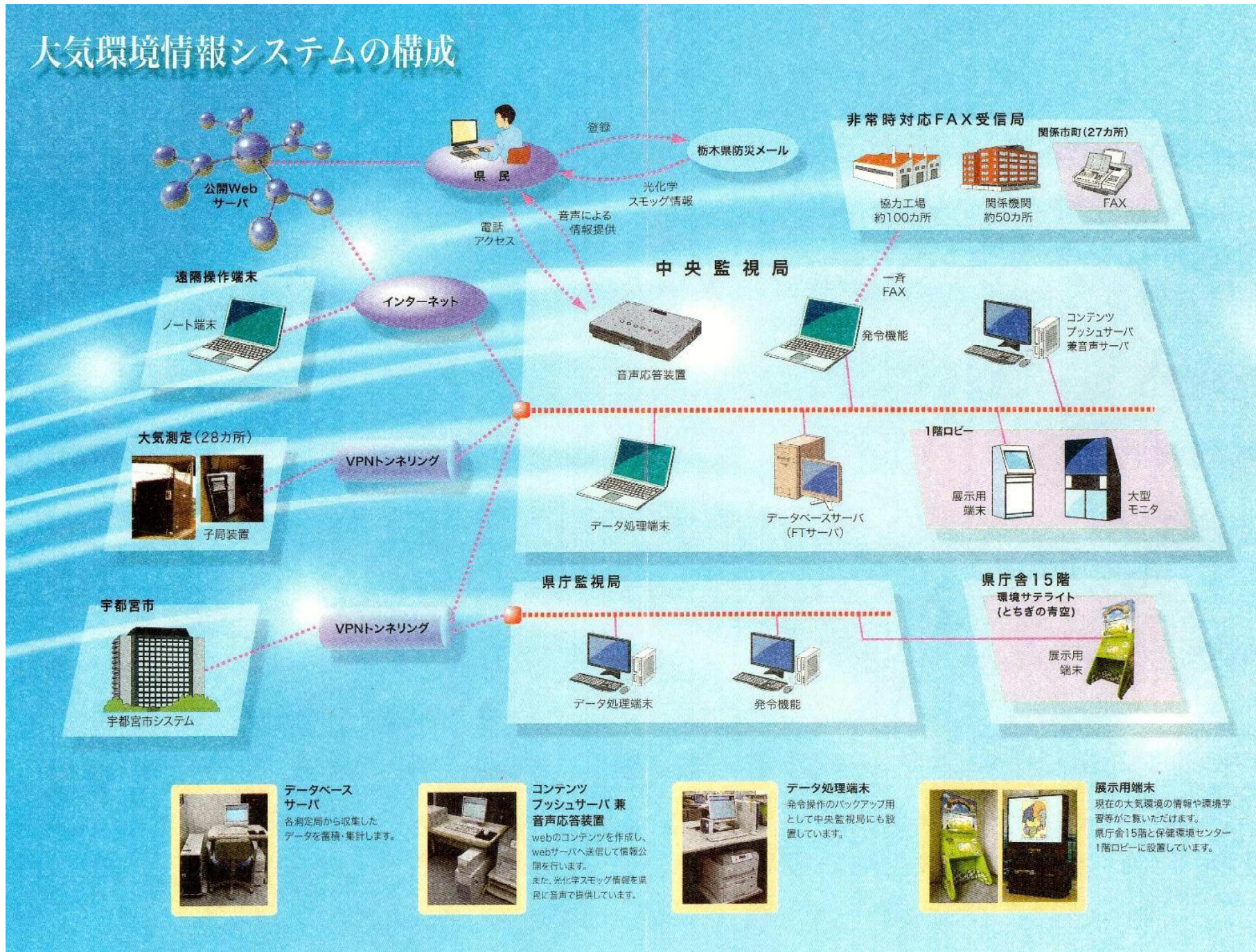
図2-2 大気環境情報システム構成図
