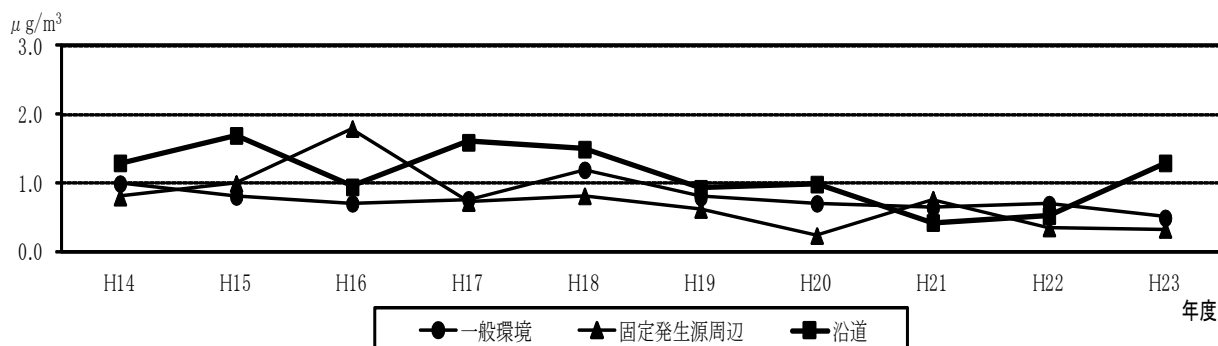
トリクロロエチレン濃度の推移〔年平均値〕
