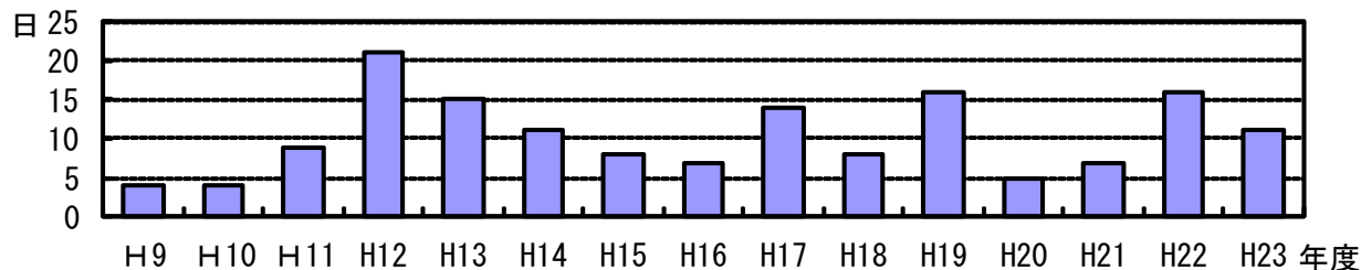
光化学スモッグ注意報発令日数の経年変化
