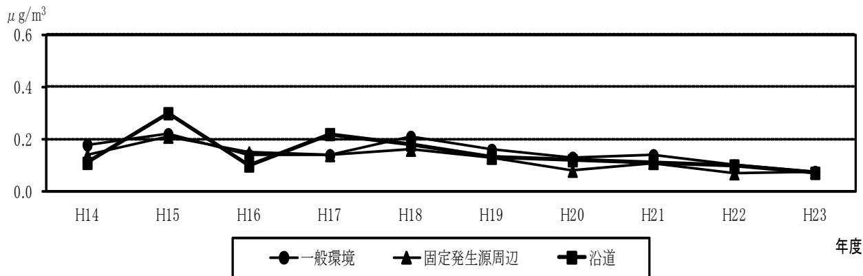
テトラクロロエチレン濃度の推移〔年平均値〕
