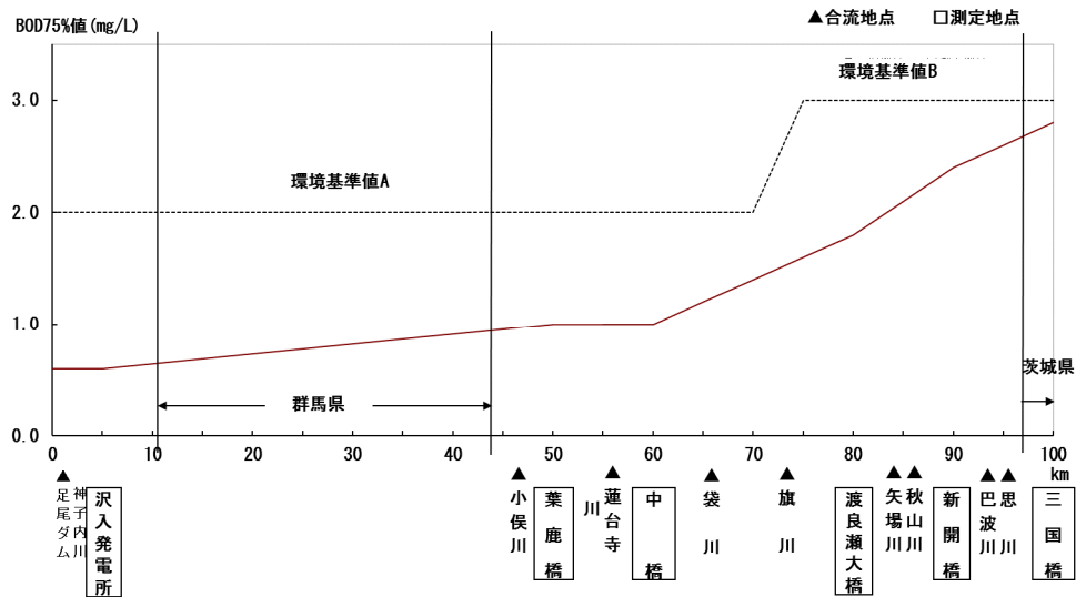
図 2-7 渡良瀬川の水質の変化（BOD75%値）
