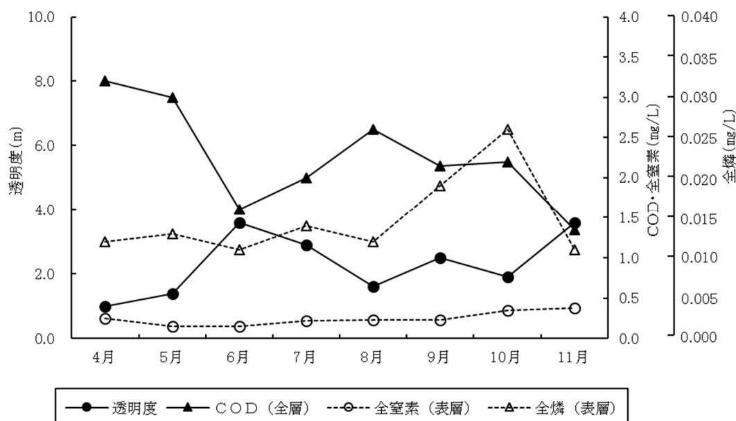
図 2-10 湯ノ湖の水質（経月変化）
