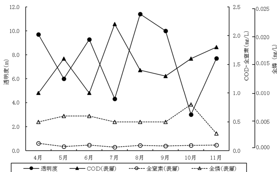
図2-9 中禅寺湖の水質（経月変化）
