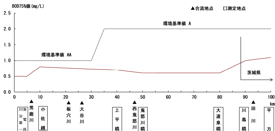
図2－6 鬼怒川の水質の変化（BOD75%値）
