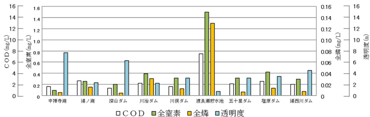
図2-11 湖沼の水質
