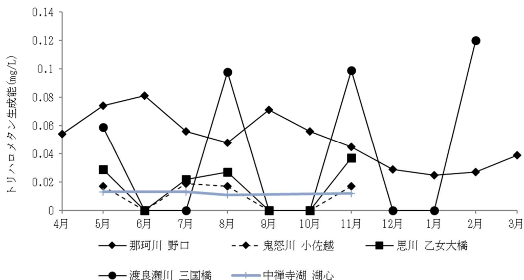
図 2-12 トリハロメタン生成能の経月変化
