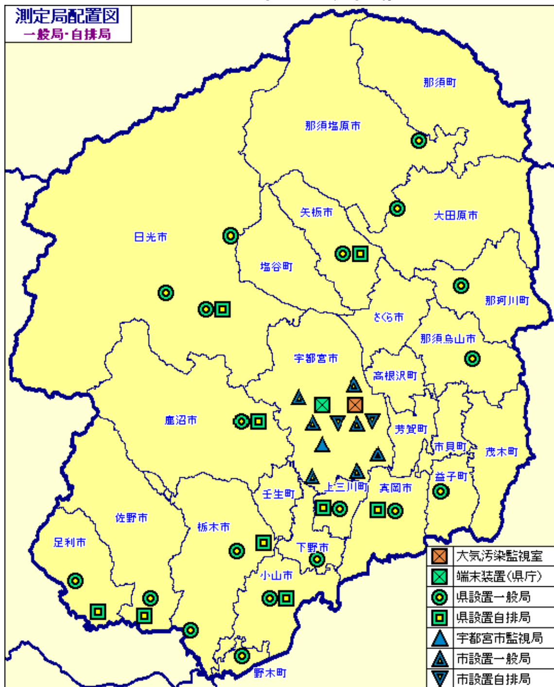
図2-1 大気汚染監視網 (平成28年3月31日現在)
