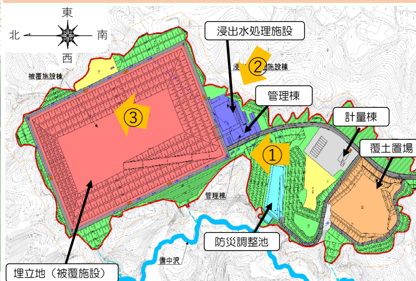
施設配置図
