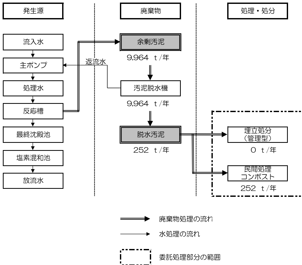
小川水処理センター廃棄物処理フロー図
