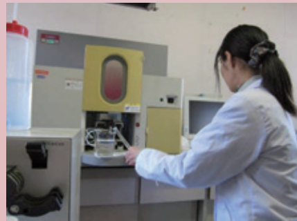
原子吸光分光光度計によりカルシウム、マグネシウム、カリウム等の肥料成分や亜鉛、銅等の有害成分を測定します。
