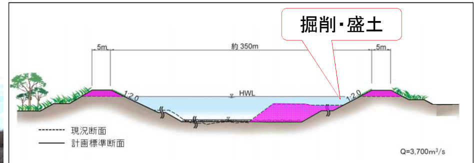
思川の河川整備イメージ
