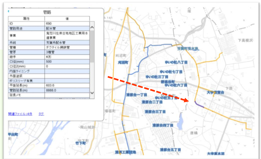
操作画面 管路敷設位置と管路情報
