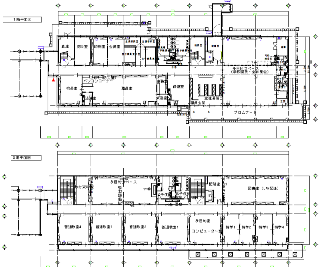
平面図
