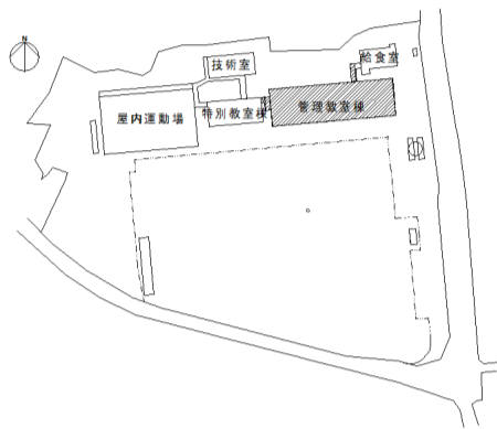
配置図
