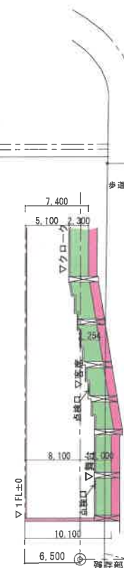
G-G' 断面図
