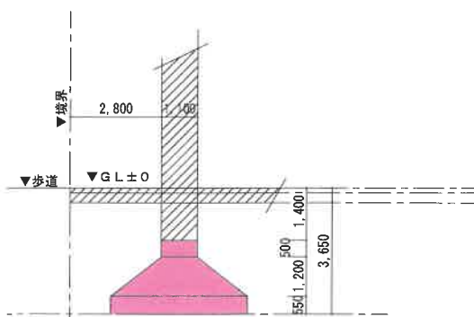
D-D' 断面図
