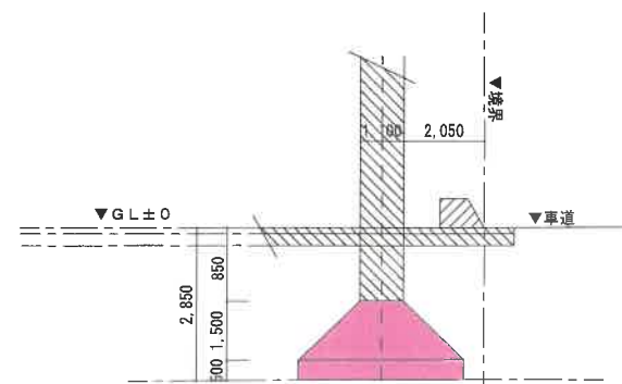
G-G' 断面図
