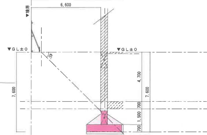
C-C' 断面図
