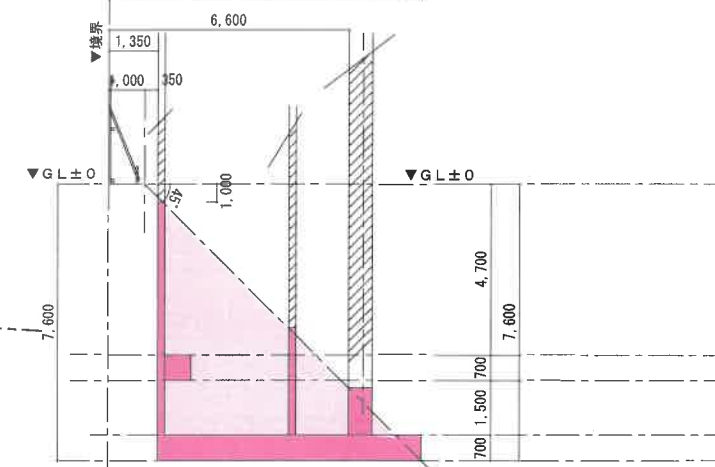
B-B' 断面図
