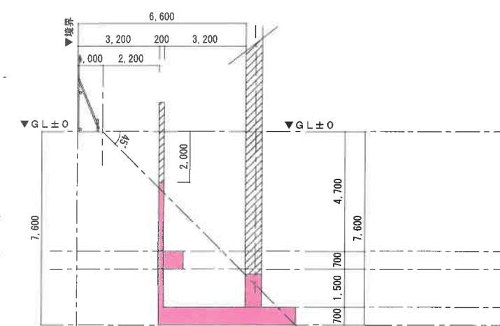
A-A' 断面図
