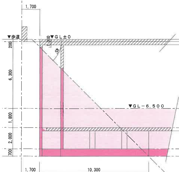
E-E' 断面図
