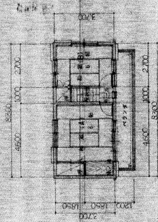
2階平面図 1:100
