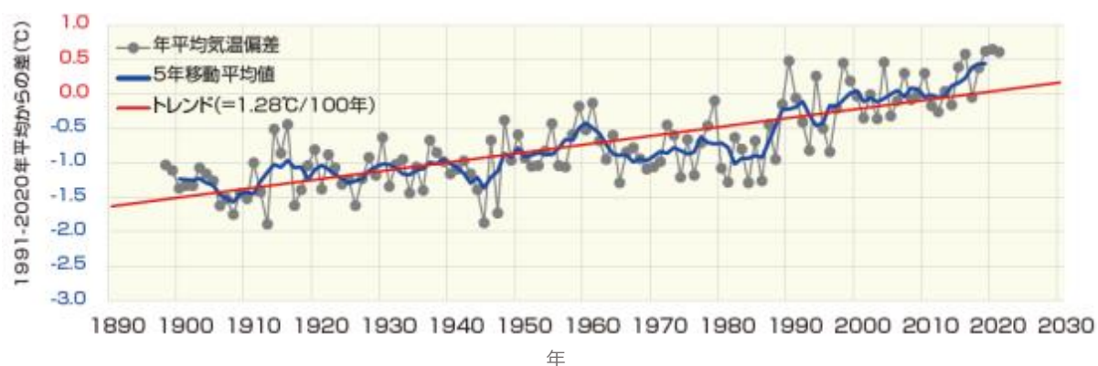
図3-2-1 日本の年平均気温偏差（1898～2021年）
