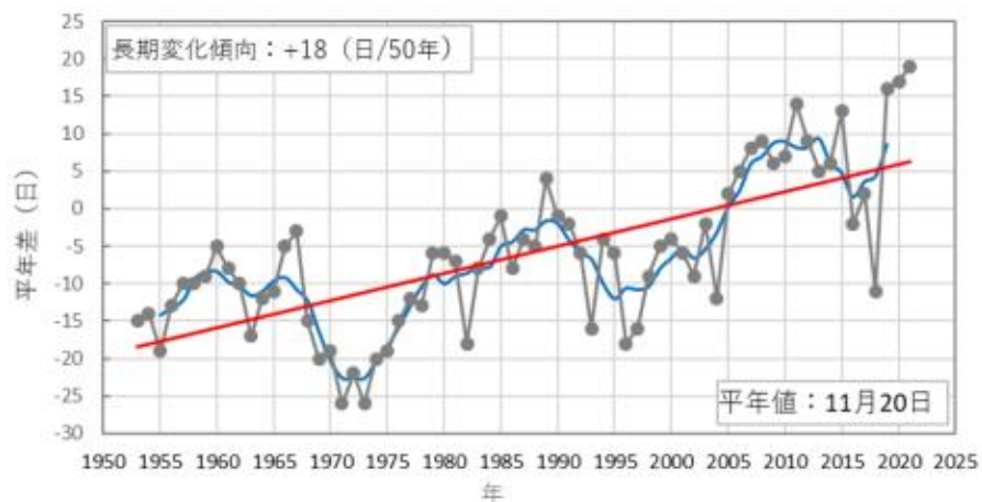
図3-2-22 紅葉日（イロハカエデ）の経年変化（宇都宮地方気象台における観測日）
