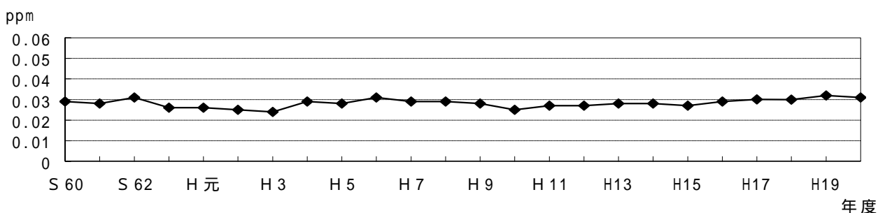
光化学オキシダント濃度の推移〔昼間の1時間値の年平均値〕
