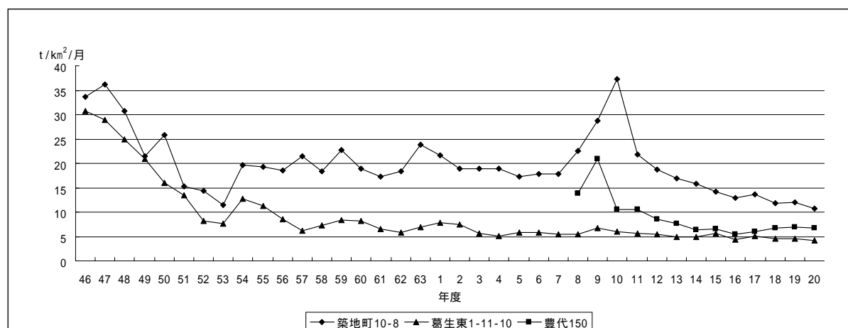
図4-1 佐野市葛生地区における降下ばいじん量の推移〔年平均値〕
