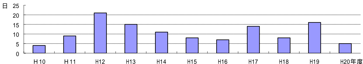
光化学スモッグ注意報発令日数の経年変化
