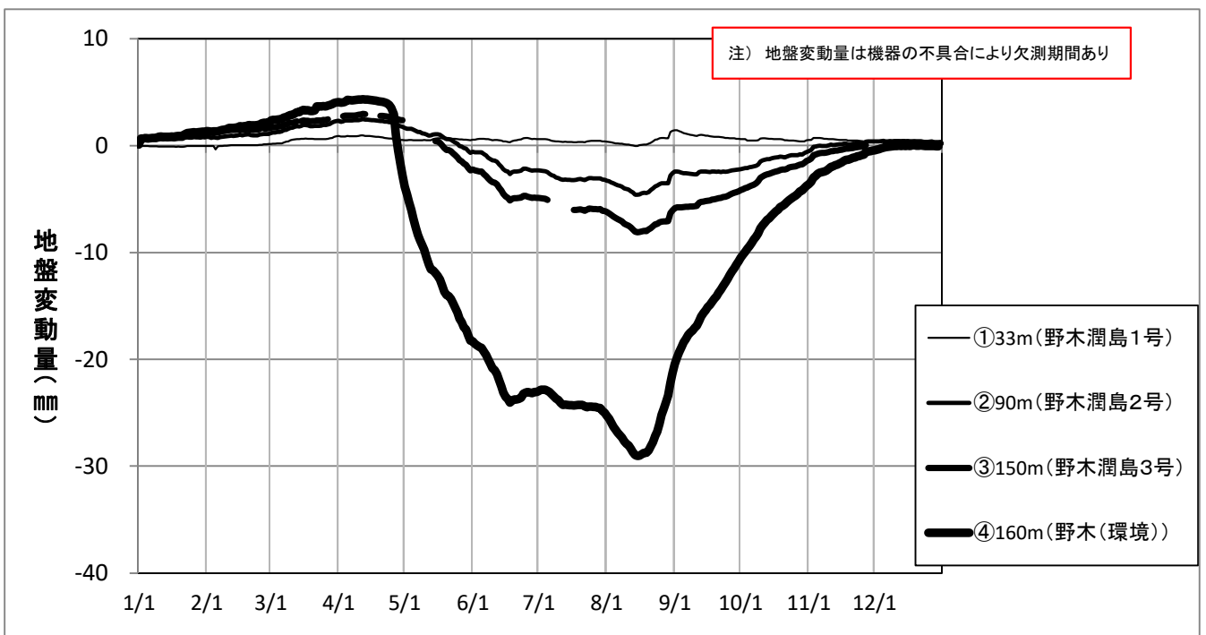
図－4 野木(環境)及び野木潤島における井戸深度別地盤変動量(令和6(2024)年)
