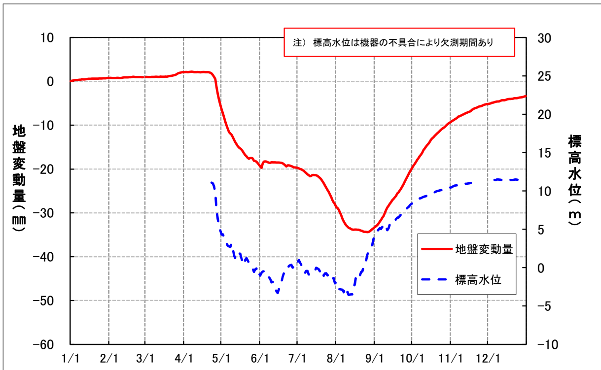
図－3 野木(環境)における地盤変動量及び地下水位状況(令和6(2024)年)
