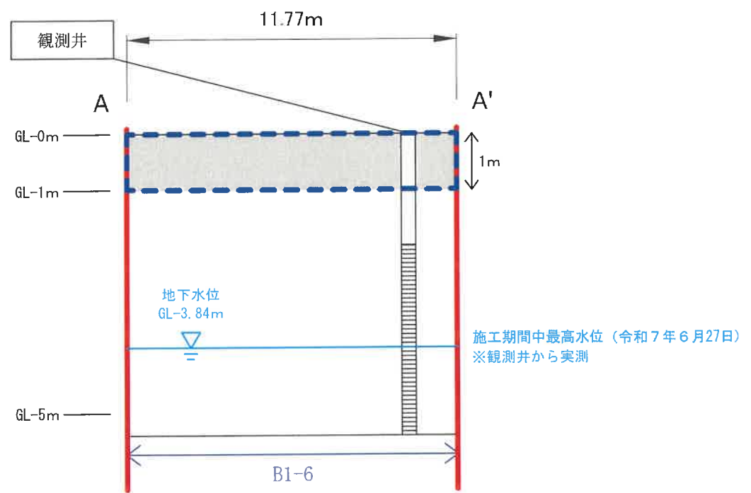
〈断面図〉
