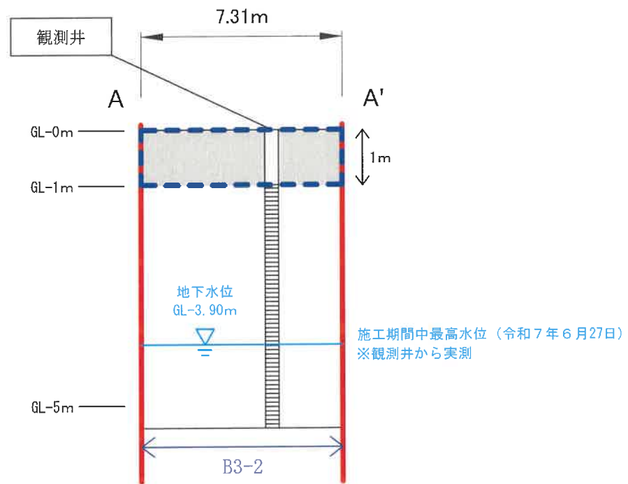
<断面図>
