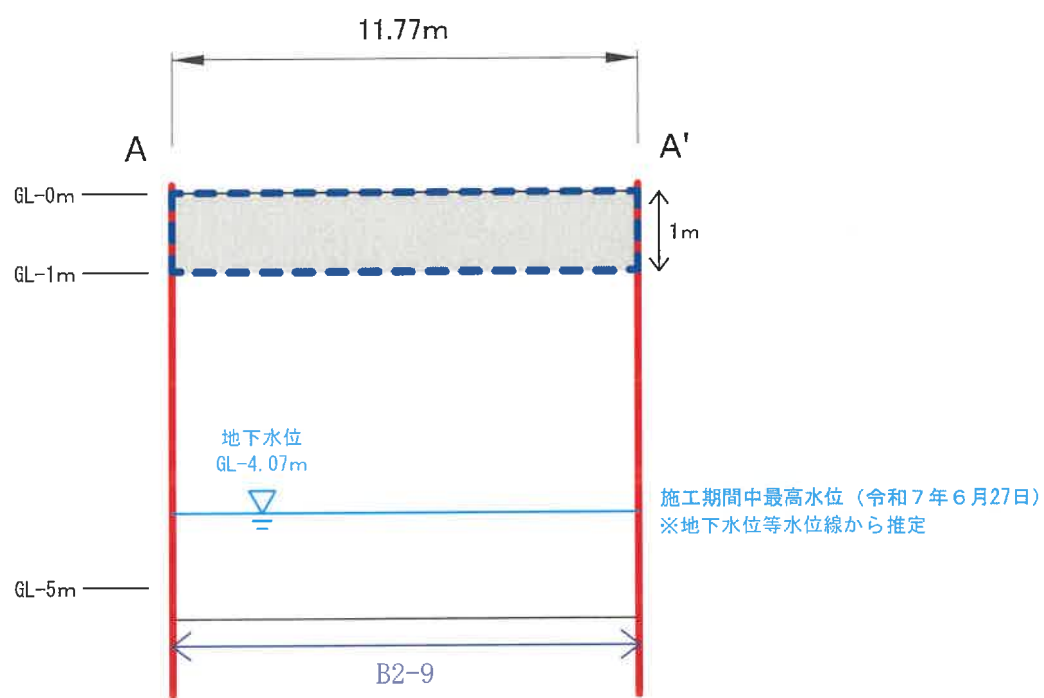
〈断面図〉
