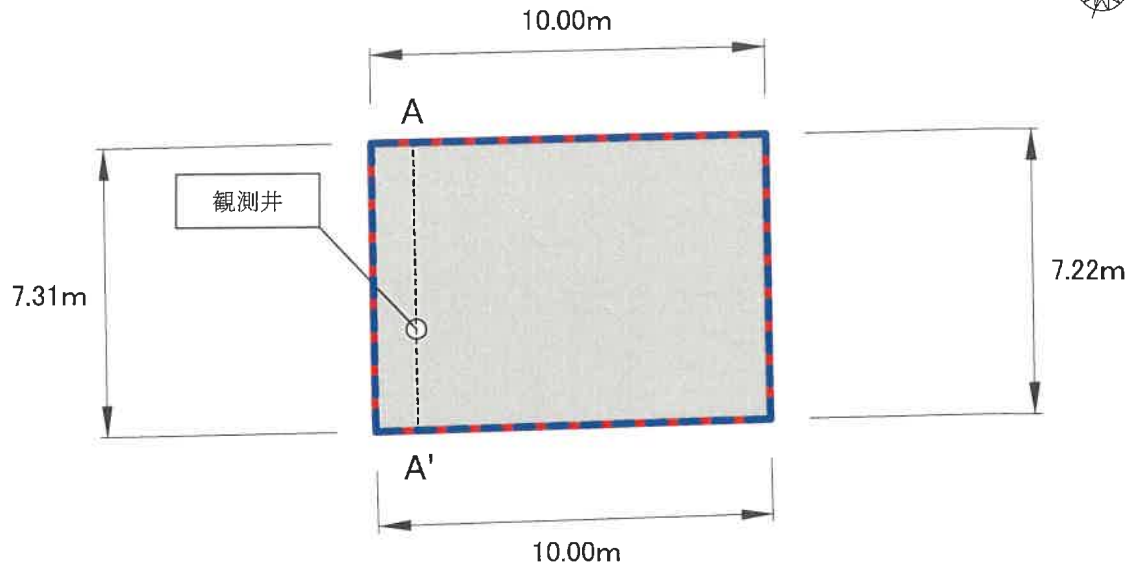
<平面図>
