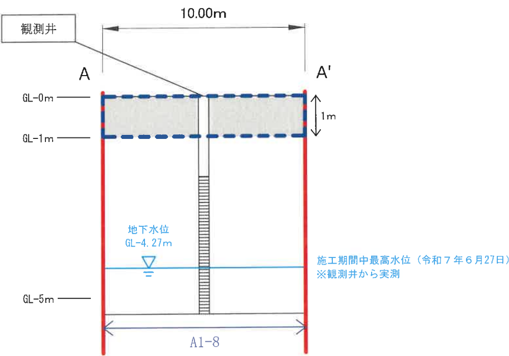
＜断面図＞
