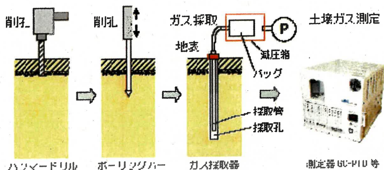
図 2. 1. 2. 1 土壌ガス調査試料採取概念図
