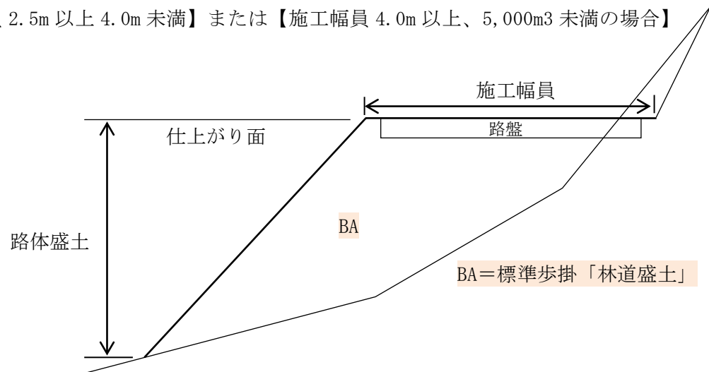
盛土積算参考図（表(a)）
