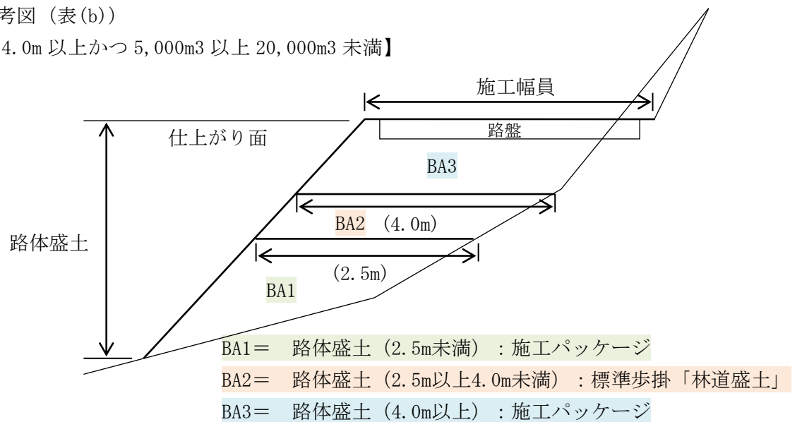
盛土積算参考図（表(c)）
