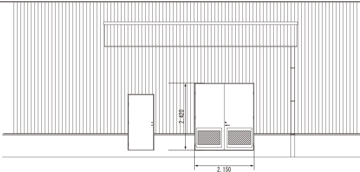
立面図
