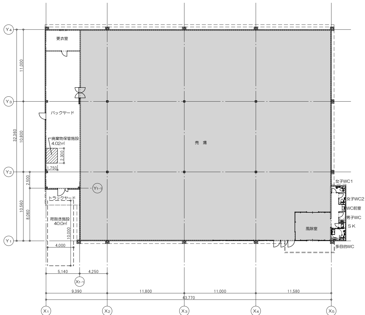
平面図
