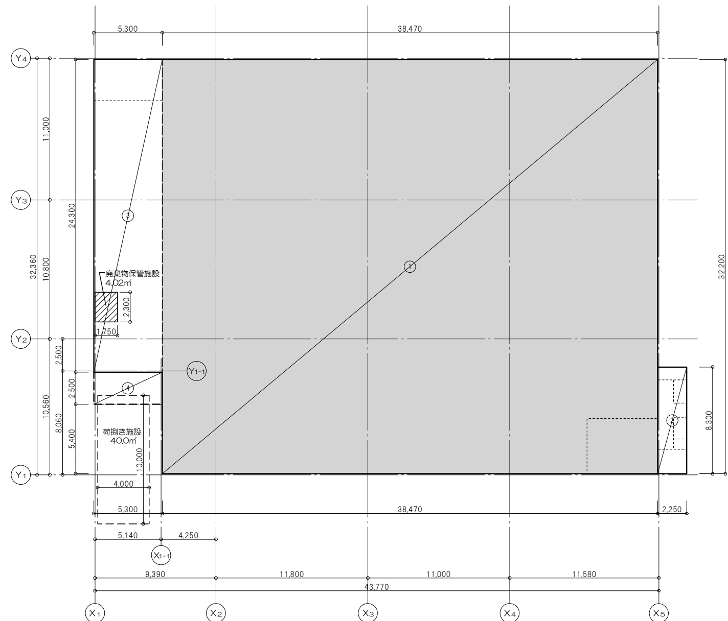
求積図
