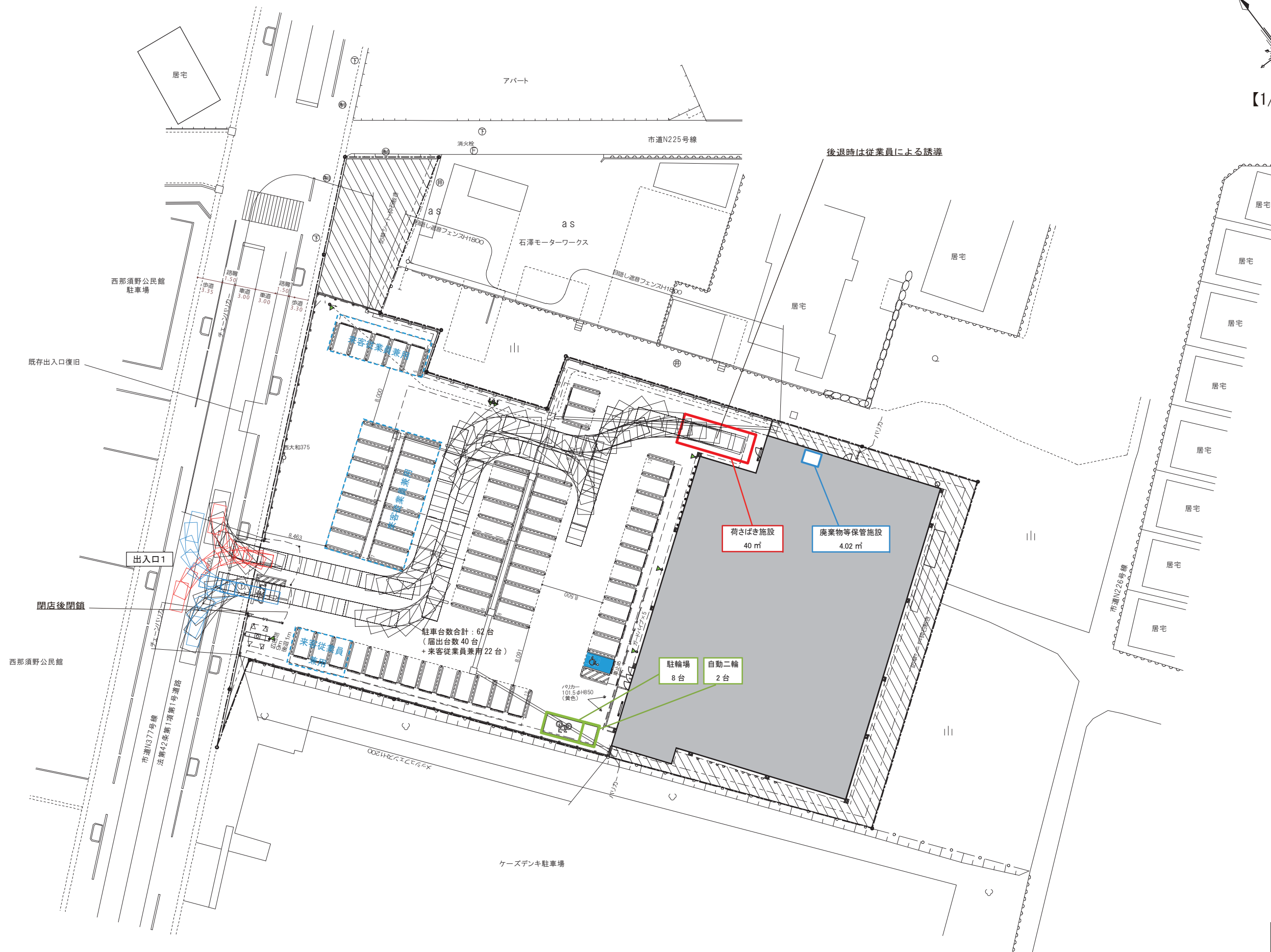
添付図 4
