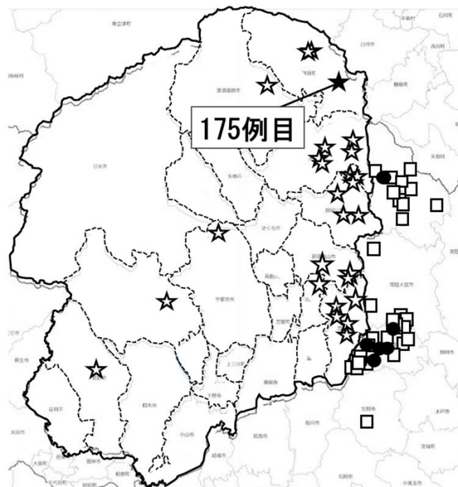
図：令和6年度以降の陽性確認地点
