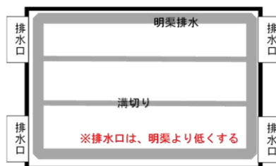
明渠排水施工のイメージ
