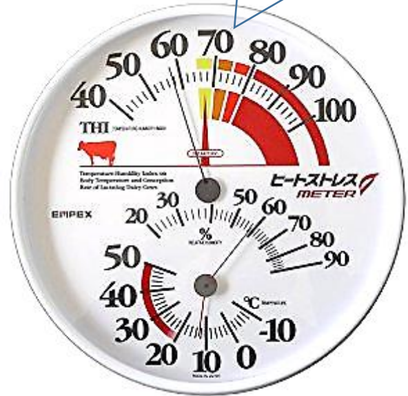
市販のヒートストレスメーター
