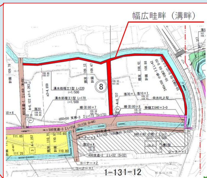
* 平面図抜粋
