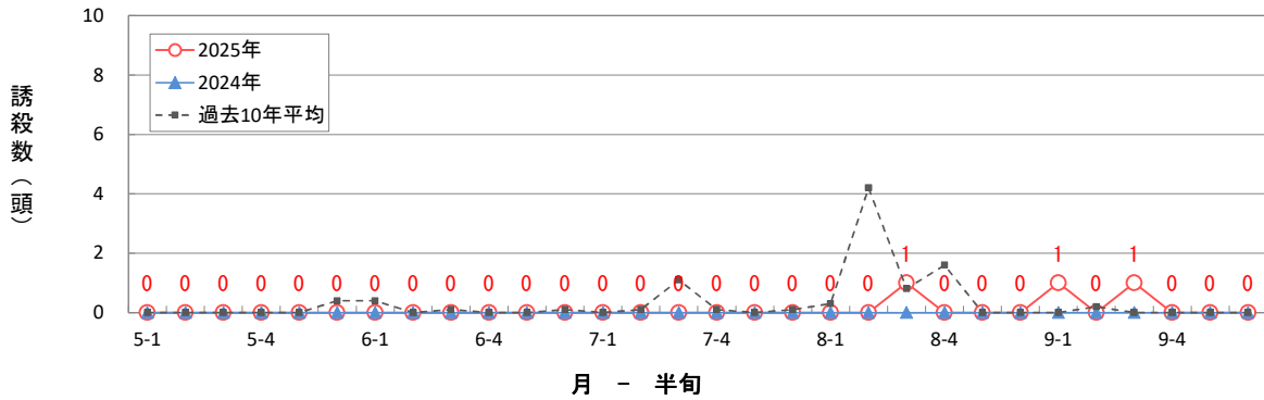
ヒメトビウンカの60W予察灯による誘殺数（小山市）
