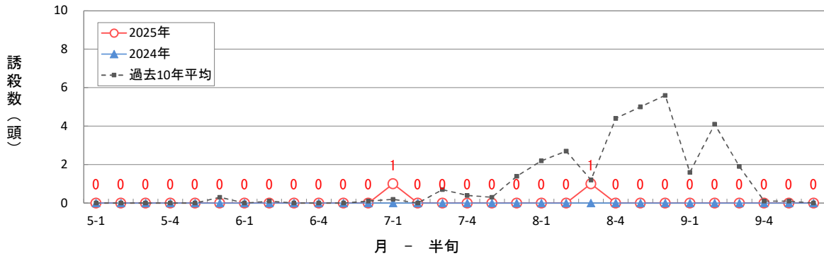
ヒメトビウンカの60W予察灯による誘殺数（栃木市大塚町）
