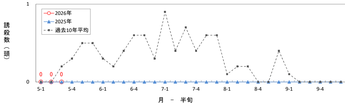
オオクロコガネの60W予察灯による誘殺数 (栃木市大塚町)
