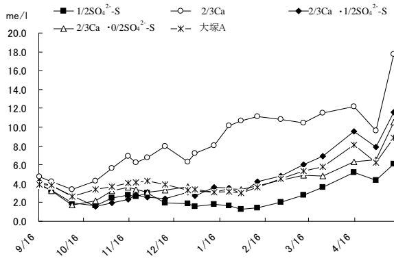
第8図 イチゴ閉鎖型養液栽培における培地内溶液 K の推移
