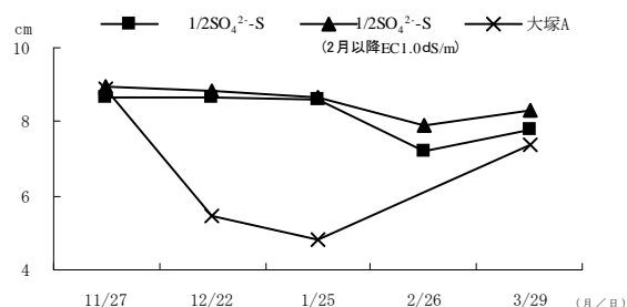
第16図 イチゴ閉鎖型養液栽培における 給液管理の違いによる葉幅の推移
