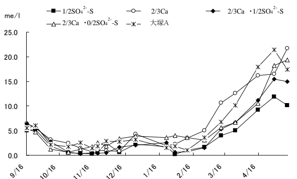
第13図 イチゴ閉鎖型養液栽培における (月/日) 培地内溶液 NO 3 -N の推移
