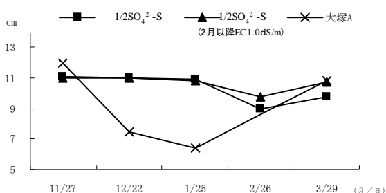
第14図 イチゴ閉鎖型養液栽培における 給液管理の違いによる葉柄長の推移
