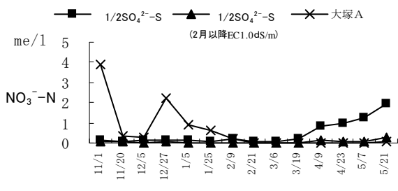
第20図 イチゴ閉鎖型養液栽培における培地内溶液 NO 3 -N の推移
