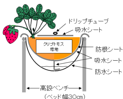
第1図 栃木県農業試験場栃木分場開発のイチゴ閉鎖型養液栽培システム
