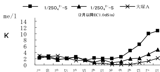
第23図 イチゴ閉鎖型養液栽培における培地内溶液 K の推移
