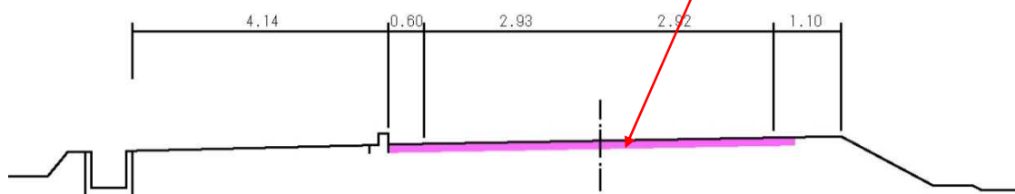
標準横断面
