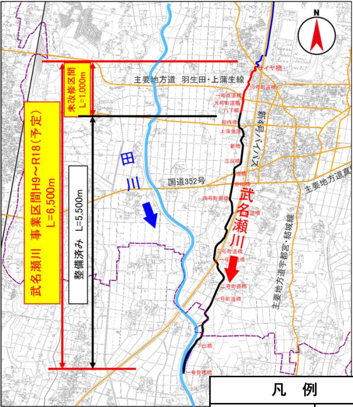
整備内容 掘削、築堤、護岸等
