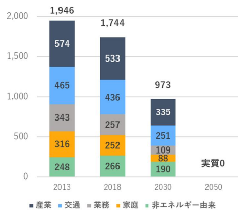
図 4-3 本県の CO 2 排出(削減)目標
