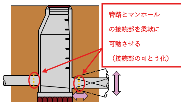
管路施設の耐震化工事
