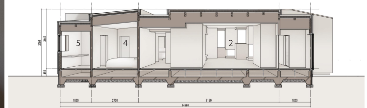
断面図 1/150
