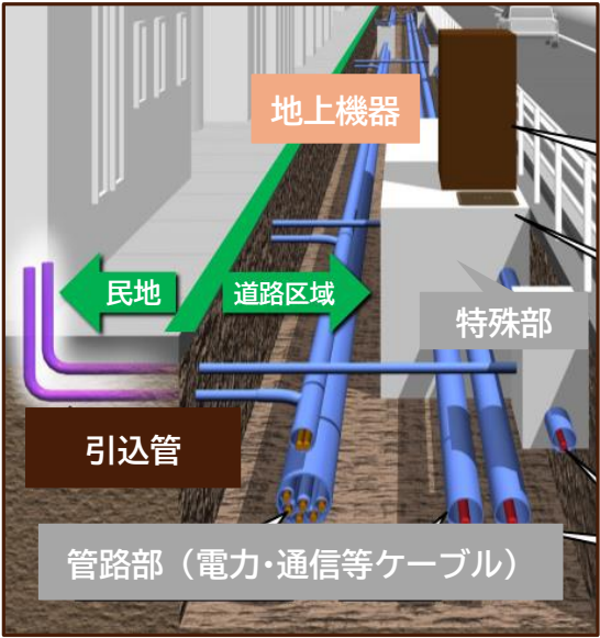
電線共同溝イメージ図
