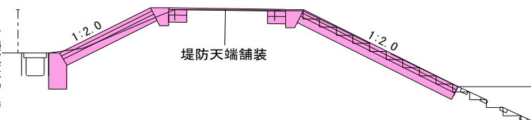
標準横断面図
