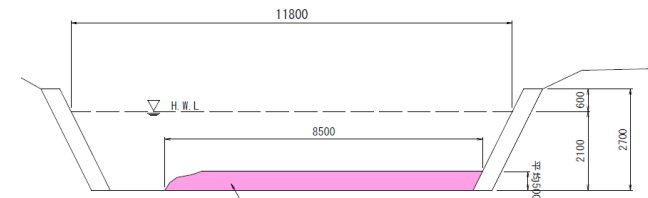
標準横断面図
