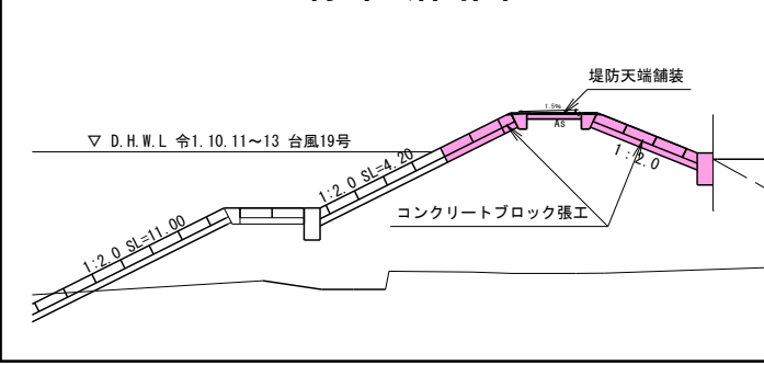
標準断面図
