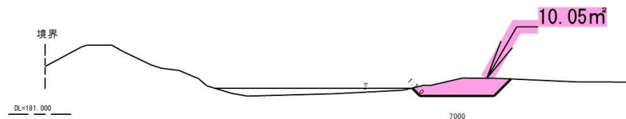
標準横断面図
