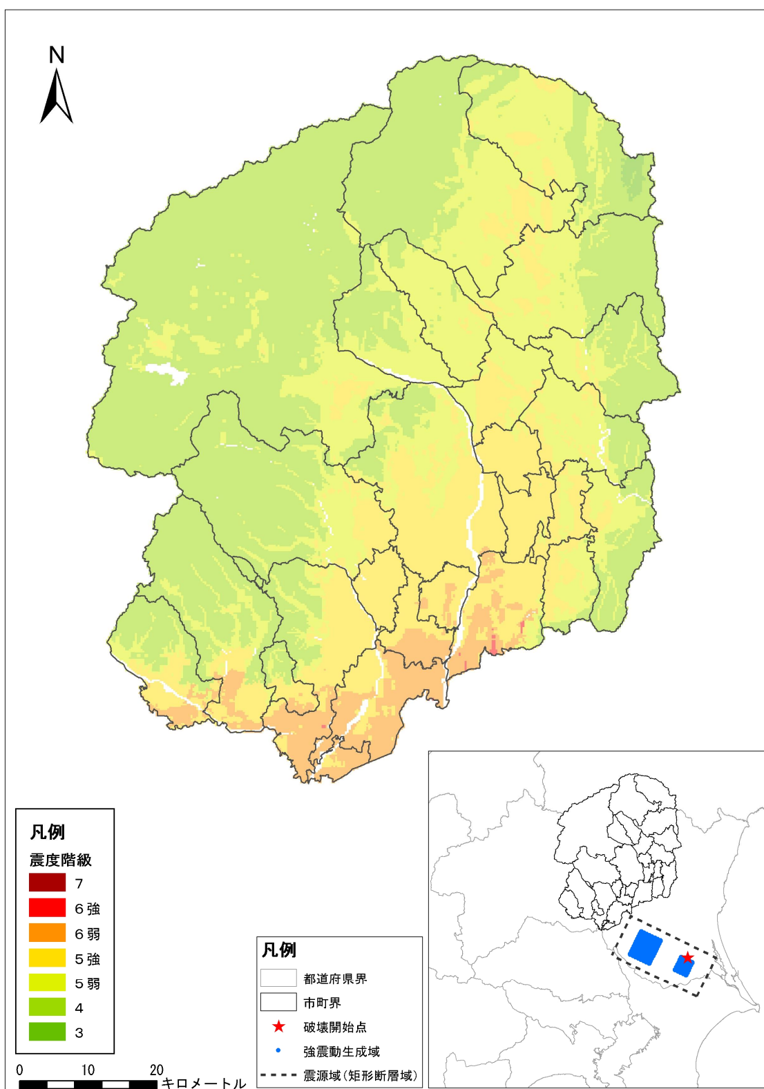
図 2.6 茨城県南西部地震（ケース 1）震度分布図
