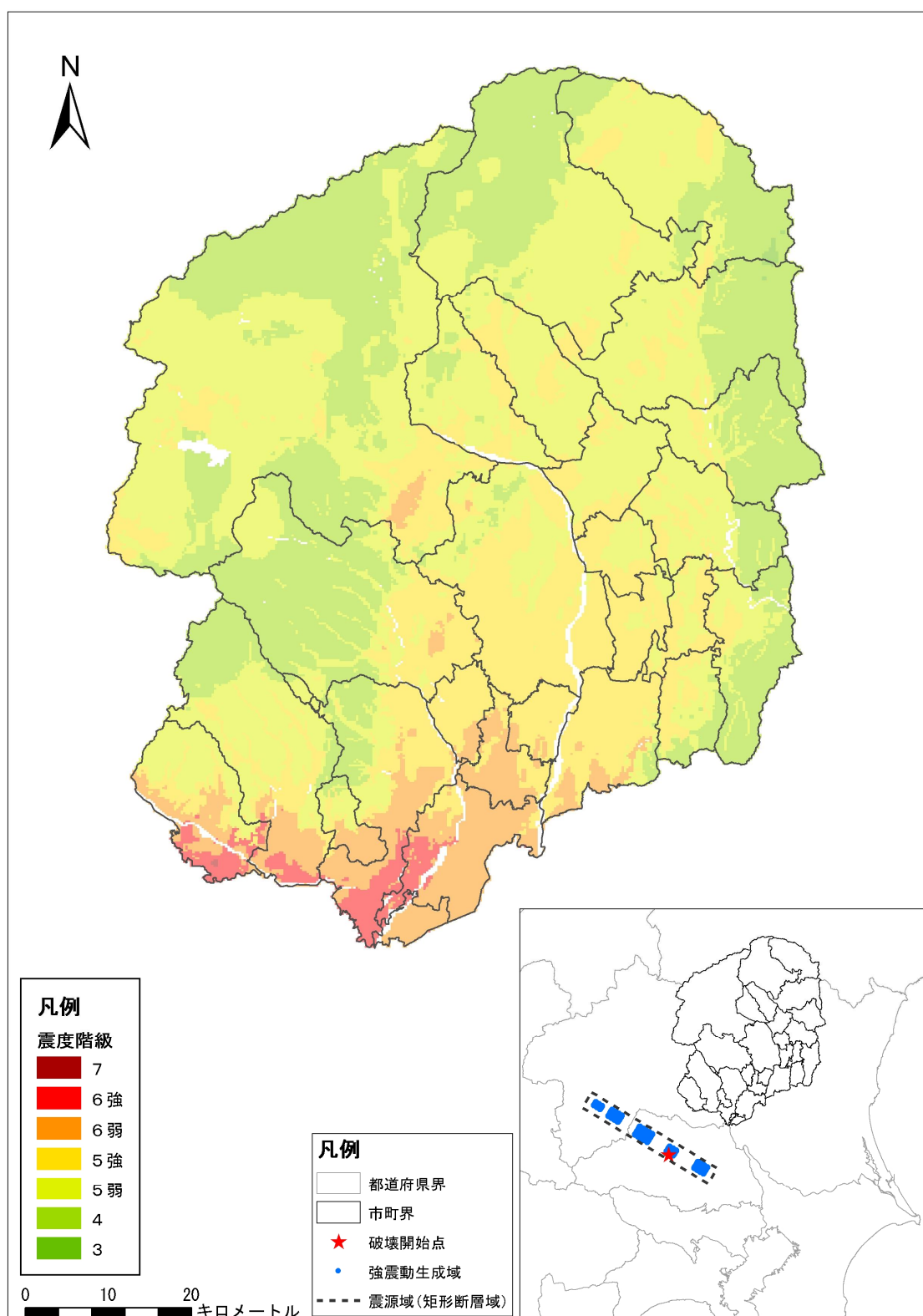
図 2.4 関東平野北西縁断層の地震（ケース 4） 震度分布図
