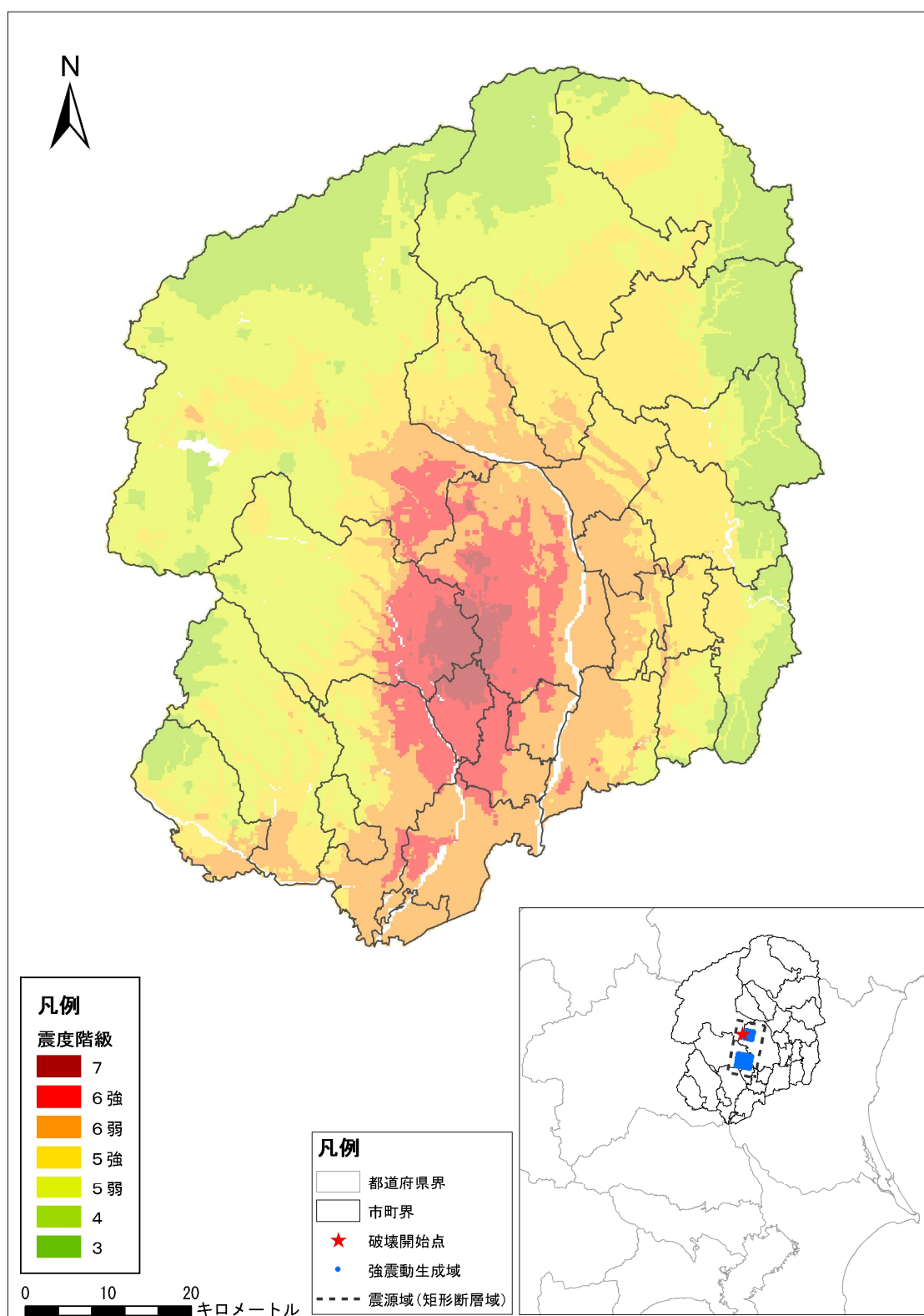
図 2.3 県庁直下に震源を仮定した地震（ケース 1）震度分布図
