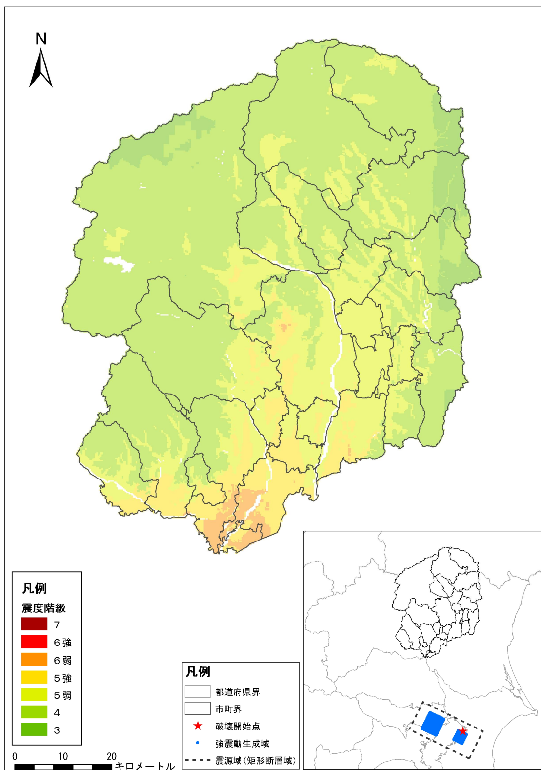
図 2.7 東京湾北部地震（ケース 1）震度分布図
