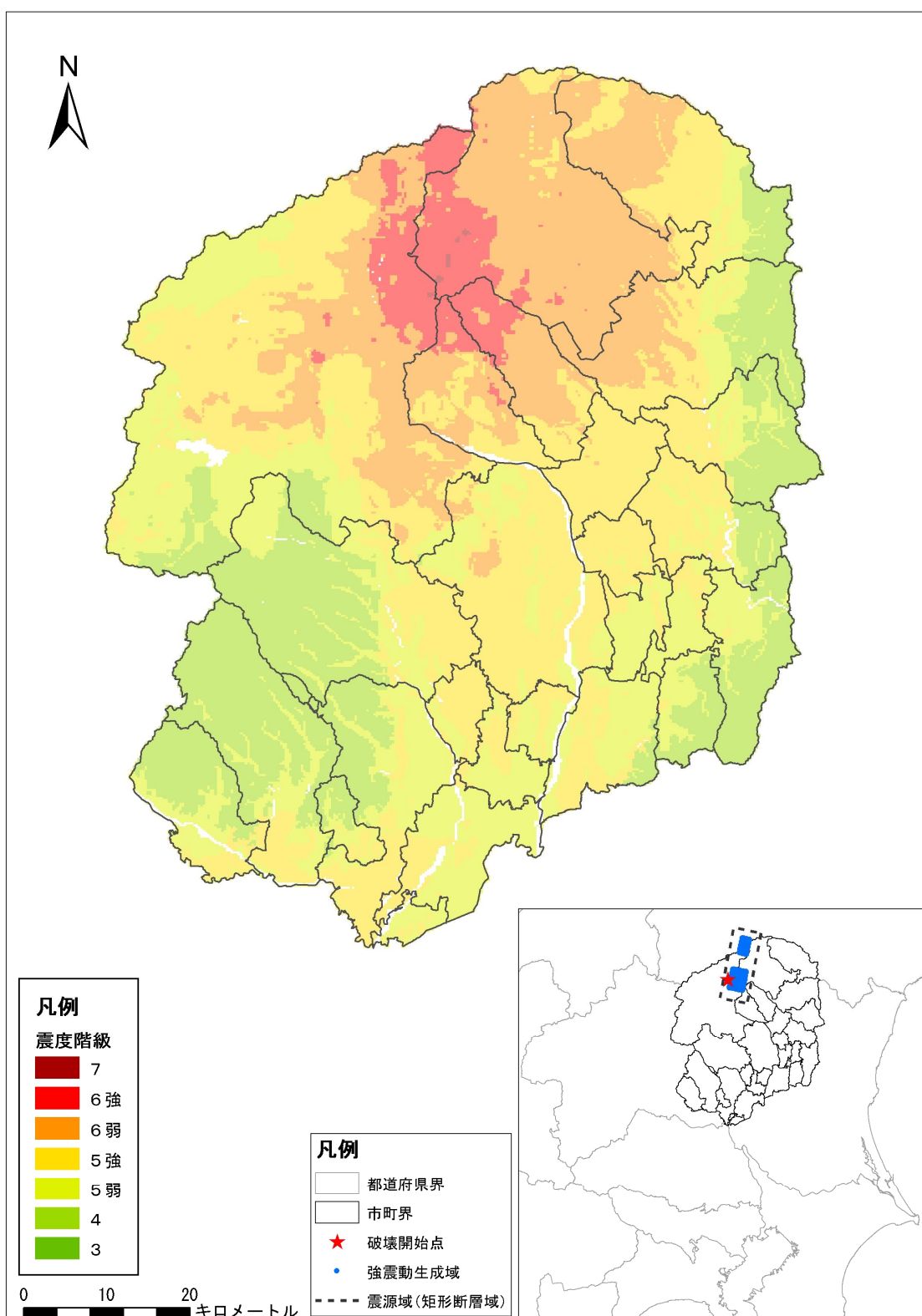
図 2.5 関谷断層の地震（ケース 1）震度分布図
