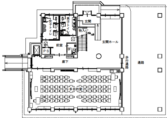
1階平面図
