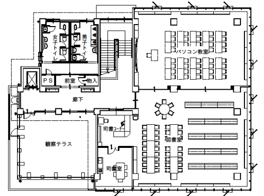
2階平面図
